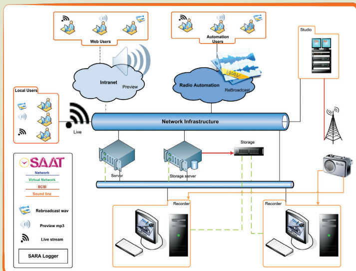
مونیتورینگ زنده ضبط شاهد
